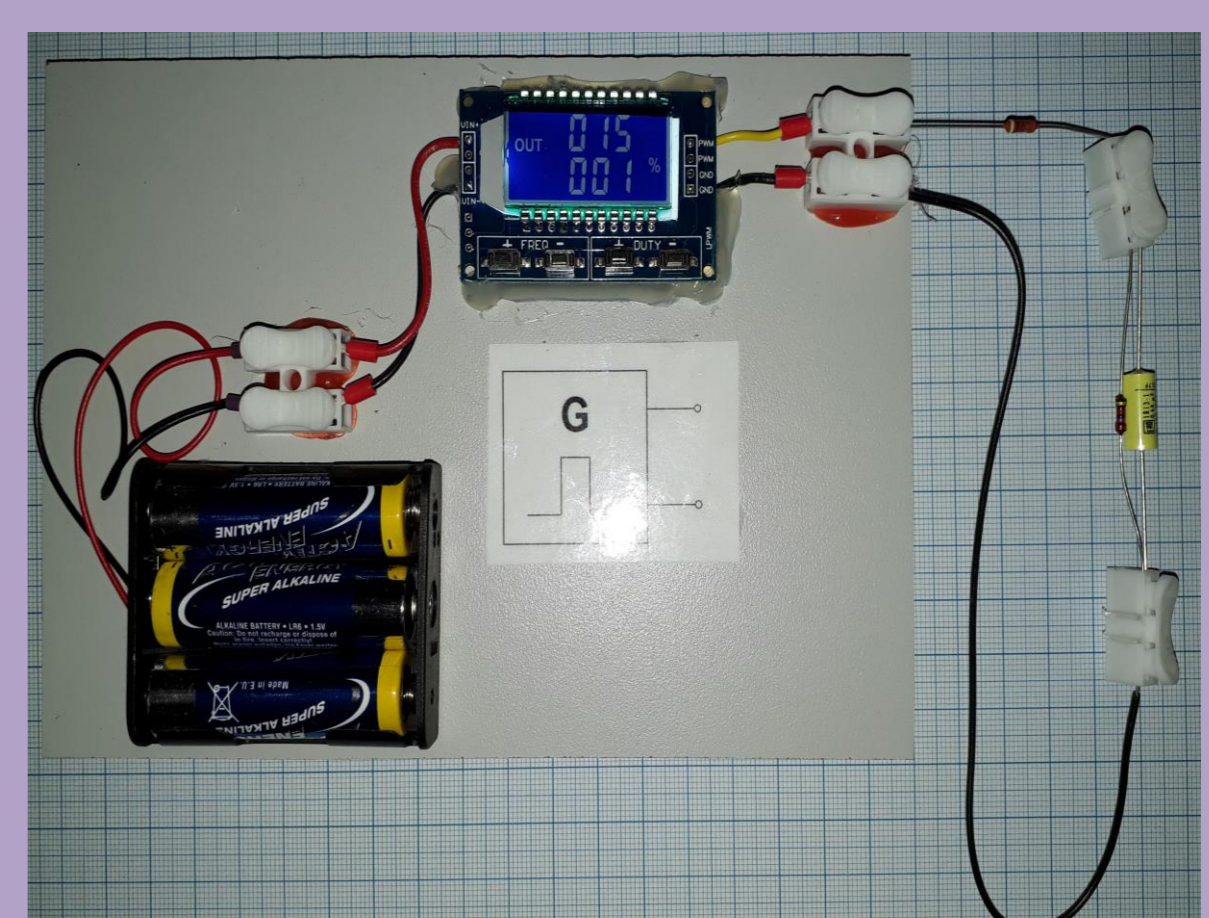
RC-Modell Biomembran
