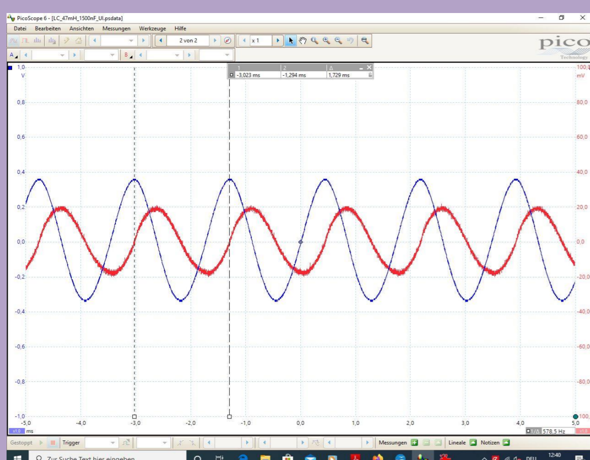
Schwingkreis
