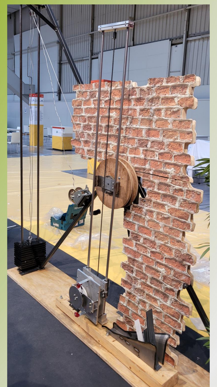
Energie-Schlitten
